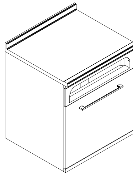
S1RS-60 L.60 P.55
