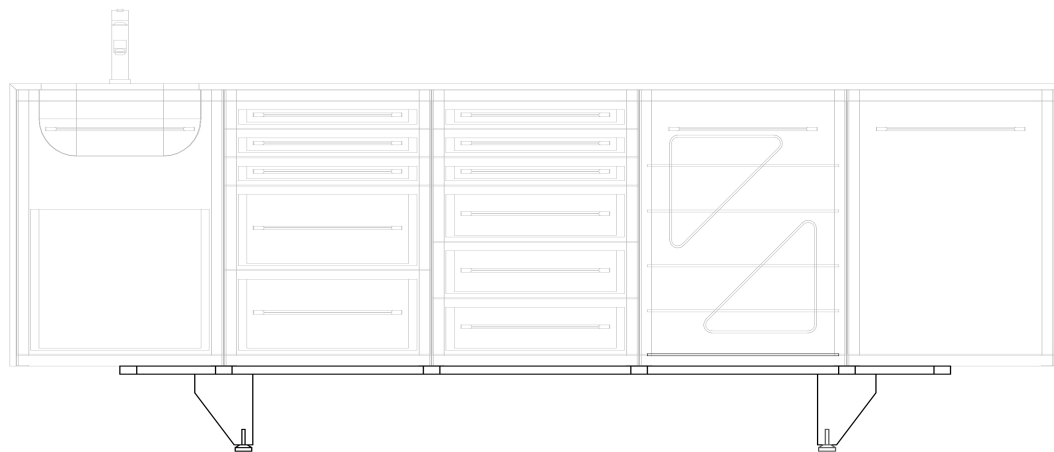
TELAIO A 5 MODULI L.2000
