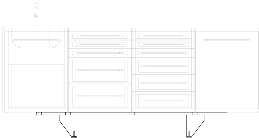
TELAIO A 4 MODULO L.1500
