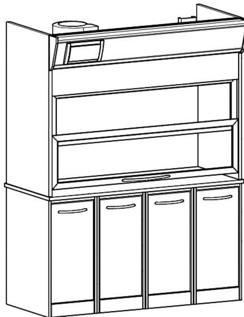
C1/A3S L.1610 H.2110 P.800
