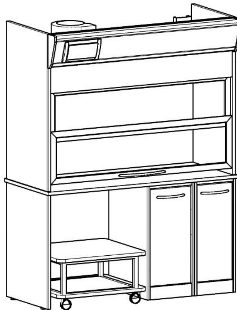
C1/RA1S L.1610 H.2110 P.800
