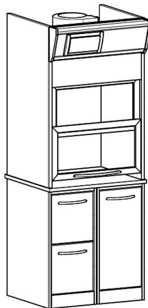
C3/C2S L.810 H.2110 P.800
