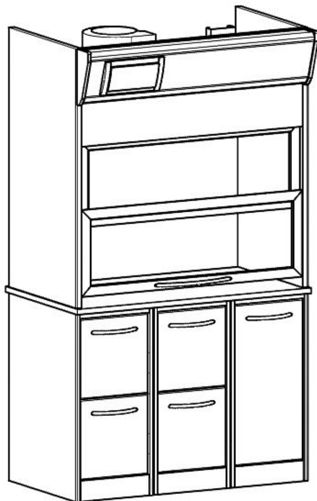
C2/C4S L.1210 H.2110 P.800
