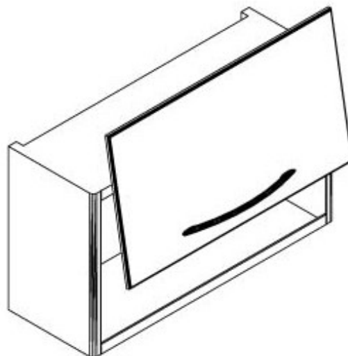
P-E1PB50 L.85 P.30
