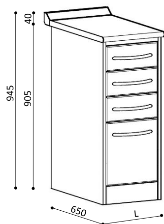
CM1-35 L.370
