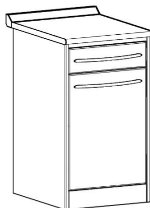
CM3-50 L.520
