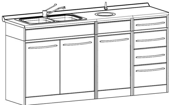
MTS2-3G/1000 L.2020 H.1000
