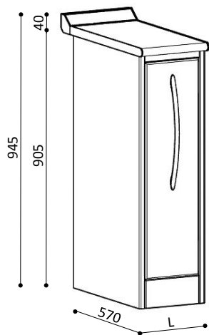
MS1/900 L.270
